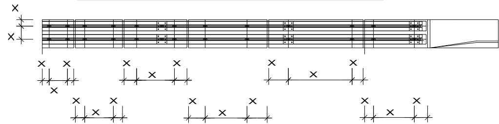
Befestigungspunkte der Schutzplanken an den Betonfertigteilen
