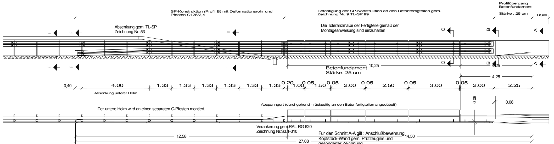
Befestigungspunkte der Schutzplanken an den Betonfertigteilen
